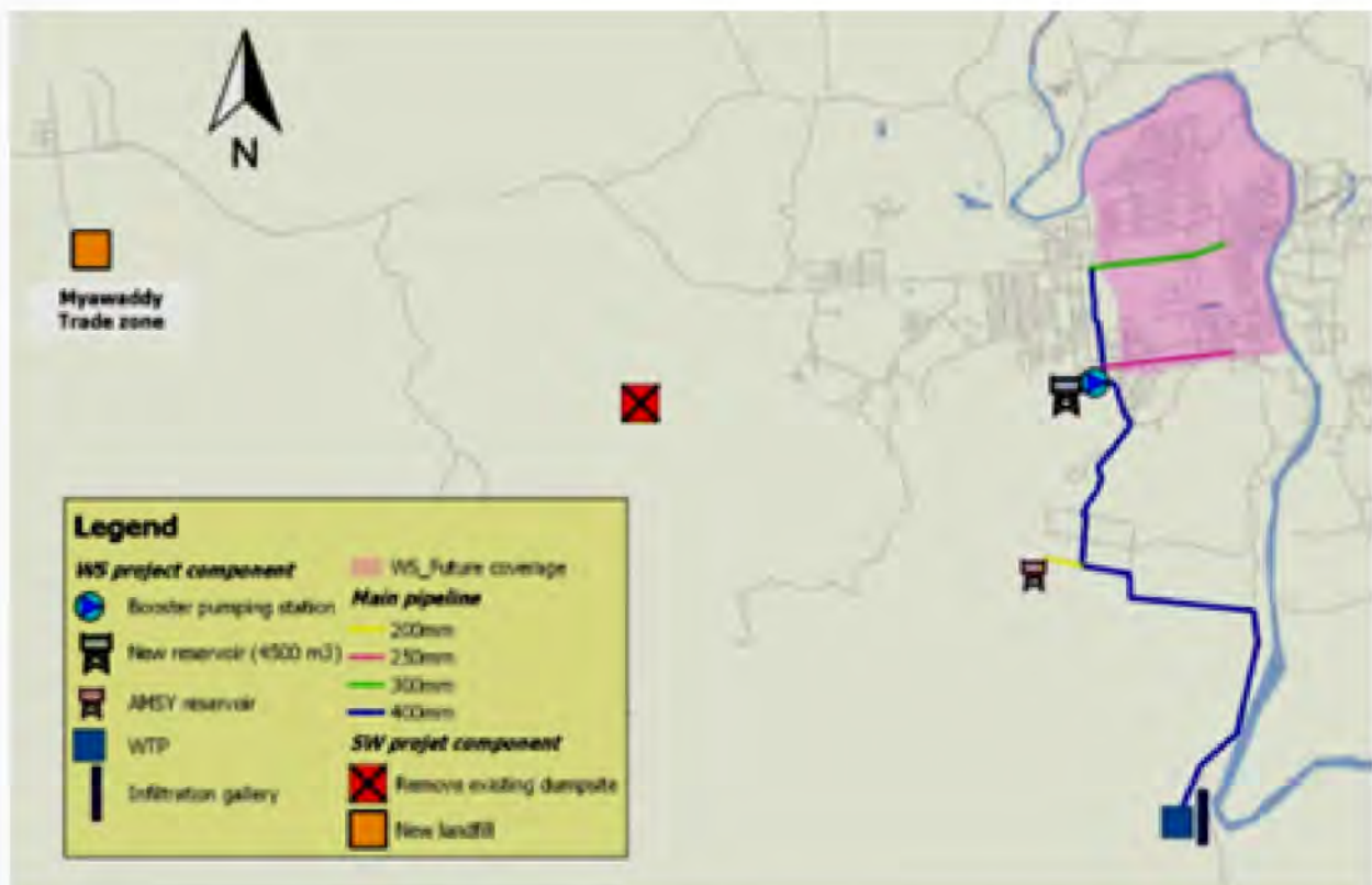
แผนที่แสดงขอบเขตการดำเนินโครงการ Corridor Towns ในส่วนของเมืองเมียวดี (ที่มา: รายงานการศึกษาความเป็นไปได้สำหรับโครงการ Third GMS Corridor Towns โดย ADB)
