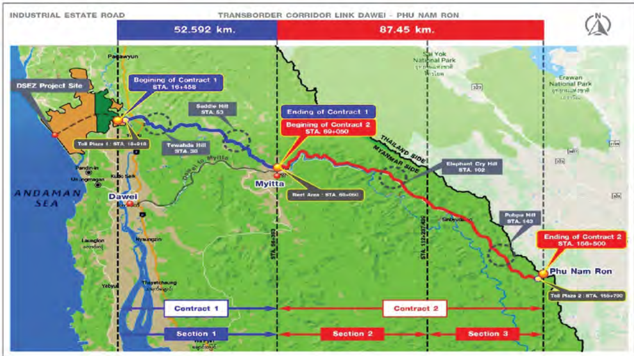
แผนที่โครงการปรับปรุงถนนสองช่องทางเชื่อมพื้นที่เขตเศรษฐกิจพิเศษชายแดนไทย-เมียนมา
